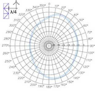
Diagrama Horizontal ajustado Lateral ¼ espaçamento
