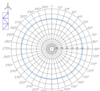
Diagrama Horizontal ajustado Lateral ¼ espaçamento
